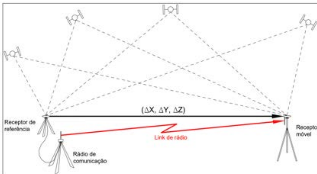
Figura 17 - RTK convencional
