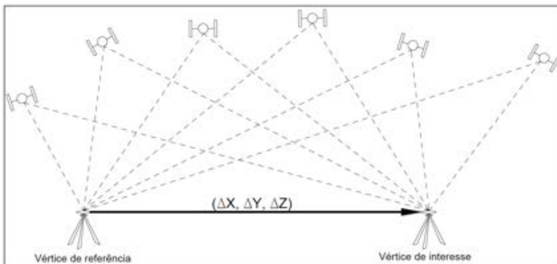
Figura 16 - Posicionamento relativo
