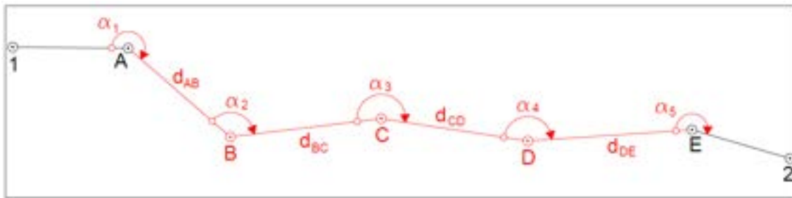
Figura 22 - Poligonal "tipo 3"
