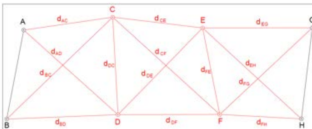
Figura 24 - Trilateração
